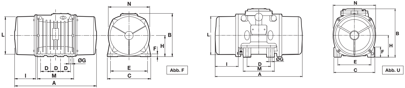
Abmessungen (mm)
