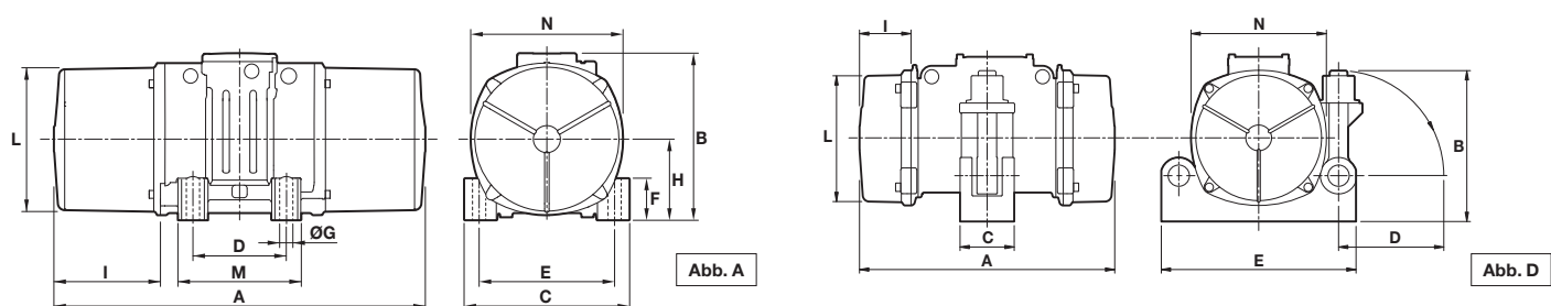
Abmessungen (mm)
