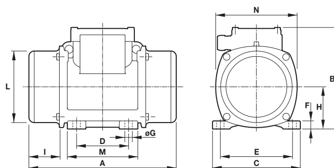
Abmessungen (mm)
